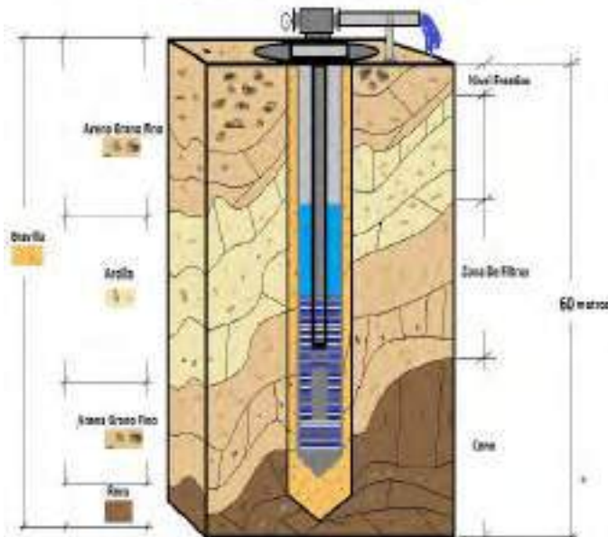
Figura 1. Perfil ilustrativo de pozo profundo.
