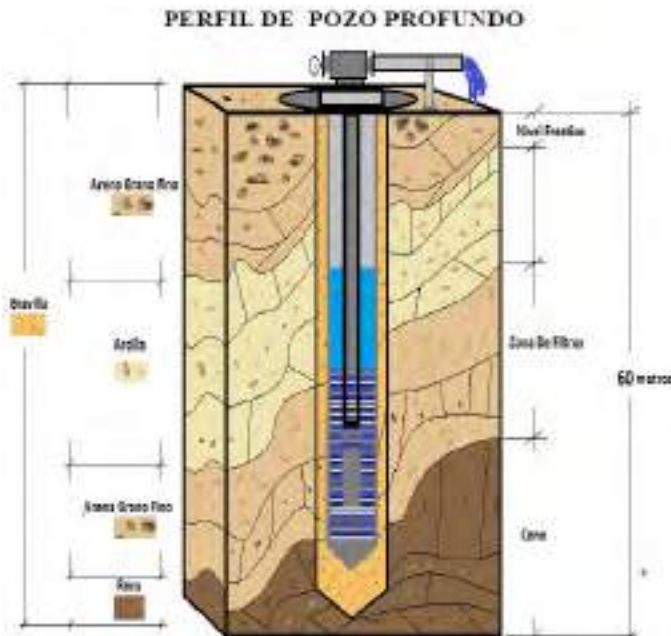
Figura 1. Perfil ilustrativo de pozo profundo.
